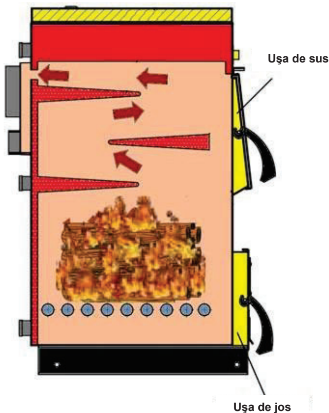
Figura 10. Verificarea clapetelor și a grilajelor cazanului
