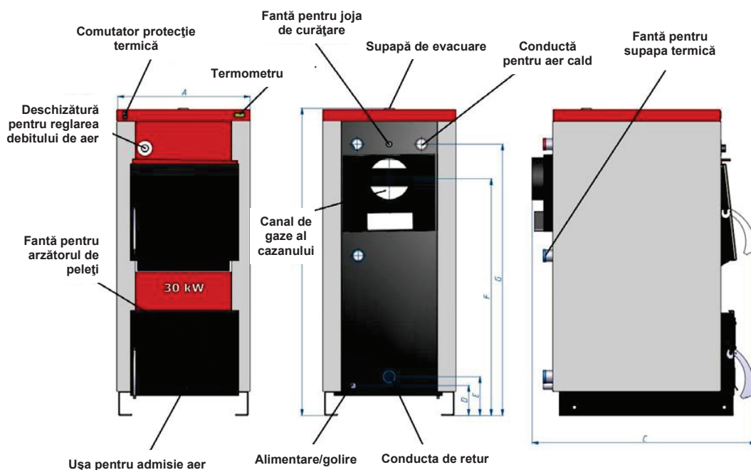
Figura 1. Dimensiuni caracteristice ale cazanelor pe combustibili solizi combinați SM
