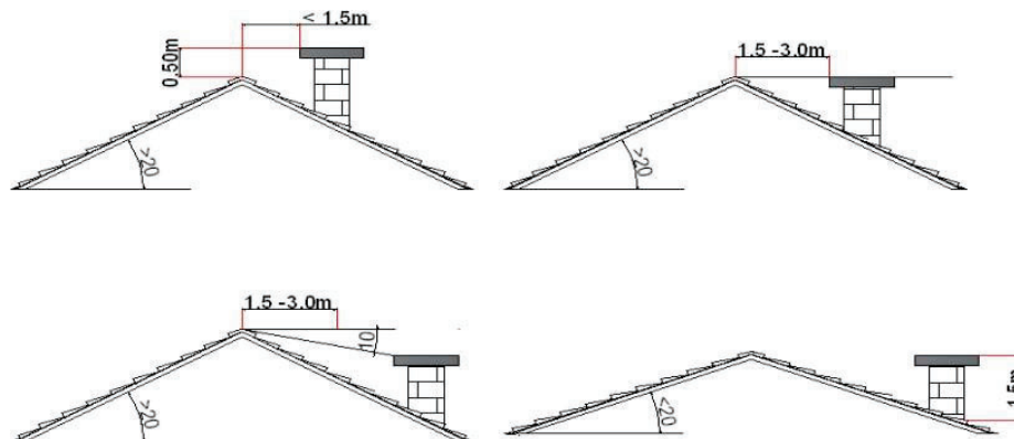
Figura 4. Amplasarea corectă a coșului de fum
