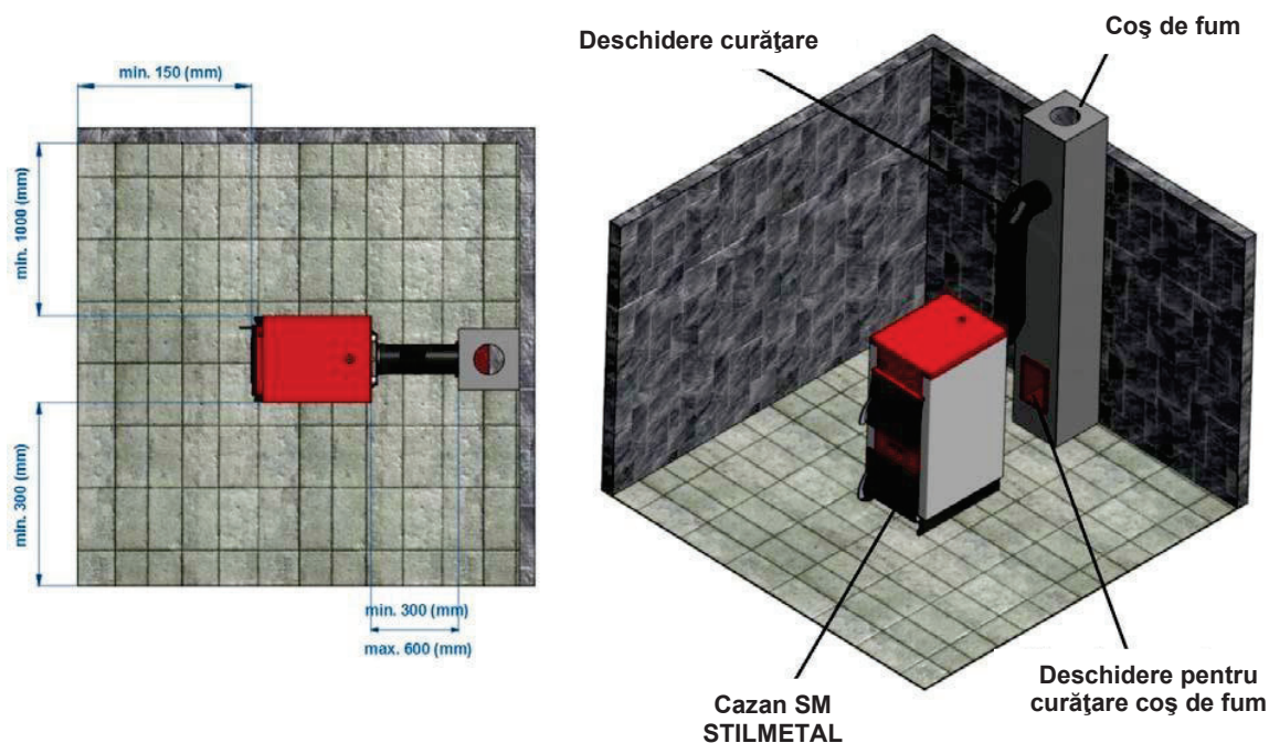
Figura 6. Amplasarea cazanului în camera tehnică
