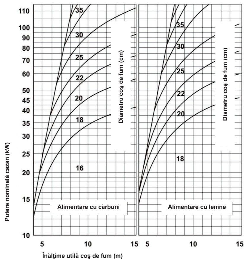
Figura 5. Dimensiunile coșului de fum pentru cazanele DOMINUS
